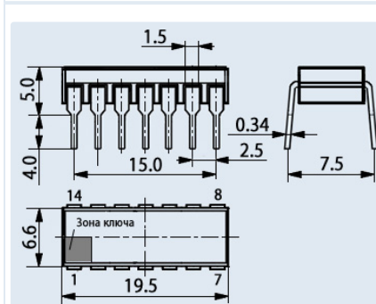
KC402A
