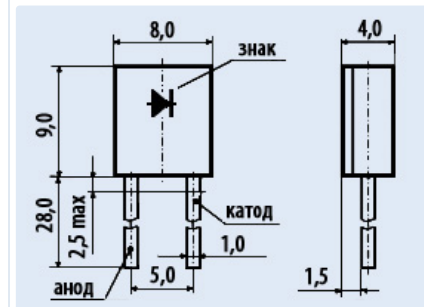
2D212A
