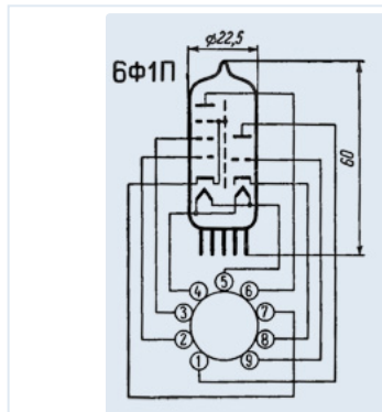
6F1P
