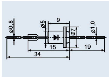
D814V
