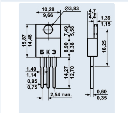
KT858A
