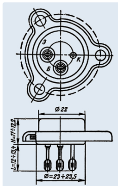
1T813B
