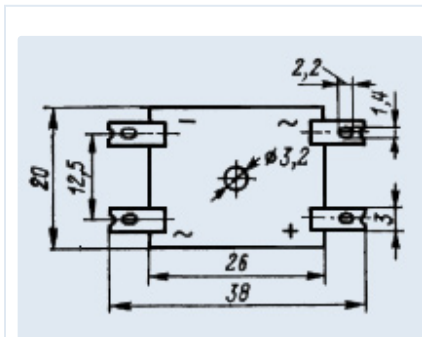
KC402A
